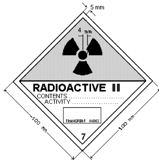
Obr. 3 Nálepka pre kategóriu II – žltá Podkladová farba hornej polovice nálepky musí byť žltá, dolná polovica biela, farba trojlístka a nápisov čierna, rímska číslica označujúca kategóriu musí byť červená.
