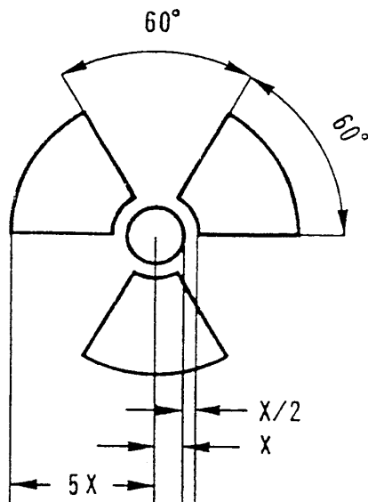
Obr. 1 Základný trojlístkový symbol s rozmermi odvodenými od priemeru stredového kruhu. Minimálna prípustná veľkosť X je 4 mm.
