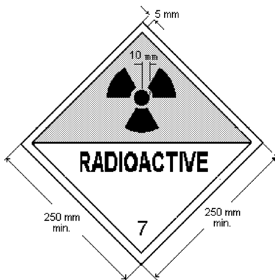
Obr. 6 Značka Minimálne rozmery sú dané; ak sú rozmery väčšie, musia byť zachované relatívne proporcie. Číslica „7“ nesmie byť menšia ako 25 mm. Podkladová farba hornej polovice značky musí byť žltá, dolná polovica biela, farba trojlístka a nápisov čierna. Použitie nápisu „Radioactive“ v dolnej polovici značky nie je povinné, čo umožňuje použiť túto značku na uvedenie príslušného kódového čísla OSN pre dodávku.
