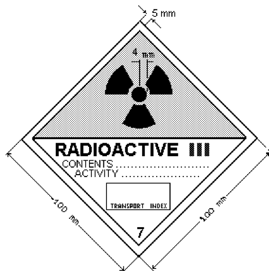
Obr. 4 Nálepka pre kategóriu III – žltá Podkladová farba hornej polovice nálepky musí byť žltá, dolná polovica biela, farba trojlístka a nápisov čierna, rímska číslica označujúca kategóriu musí byť červená.
