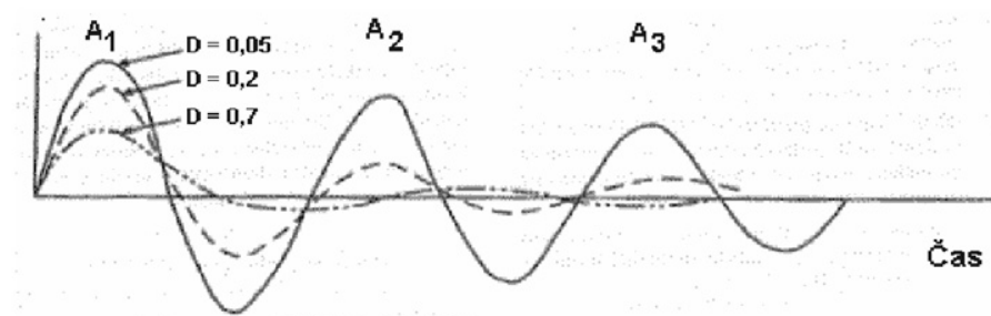
Tlmený prechodový jav
