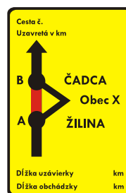
IS 16 Návesť pred obchádzkou (odklonom)
