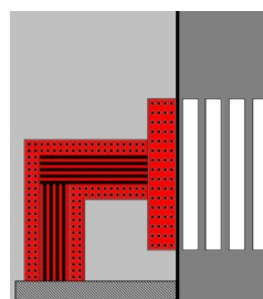
Z 8c Signálny pás pre nevidiacich na chodníku pred priechodom pre chodcov
