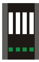
V 7a Priechod pre cyklistov prímknutý k priechodu pre chodcov
