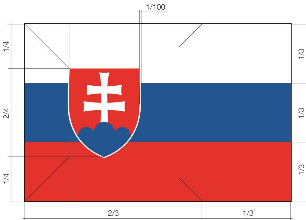
Štátna vlajka Slovenskej republiky – zostavovací nákras
