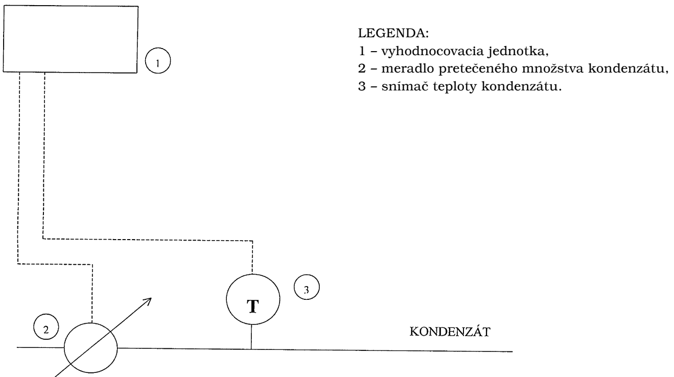
Obrázok č. 3: Metóda merania tepla v kondenzáte.
